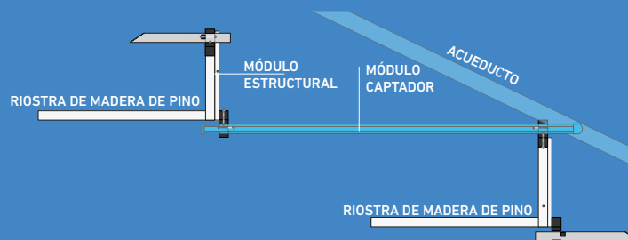
DETALLE ESTRUCTURA DE ATRAPANIEBLAS ELEVACIÓN FRONTAL Y PLANTA DE MODULO ESTRUCTURAL
