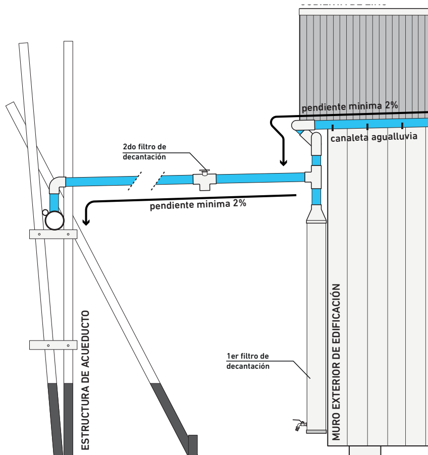
ESQUEMA ENERGÍA /GRAVEDAD POR INCLINACIÓN
