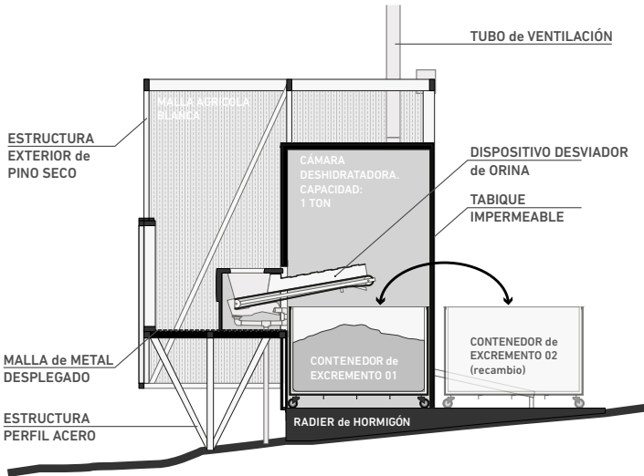
DETALLE BAÑO SECO
